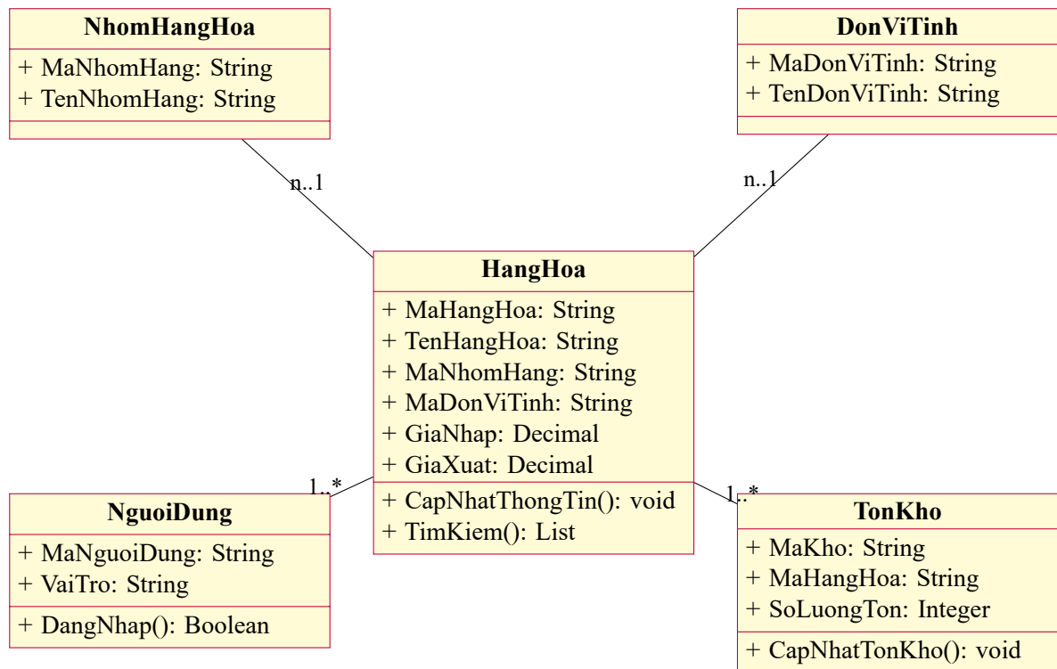
Hình 4.5: Biểu đồ lớp trong ca sử dụng UC13 – Thêm hàng hóa
