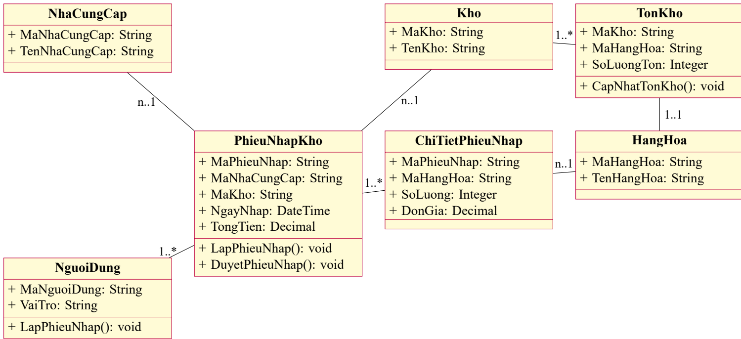
Hình 4.6: Biểu đồ lớp trong ca sử dụng UC23 – Lập phiếu nhập kho
