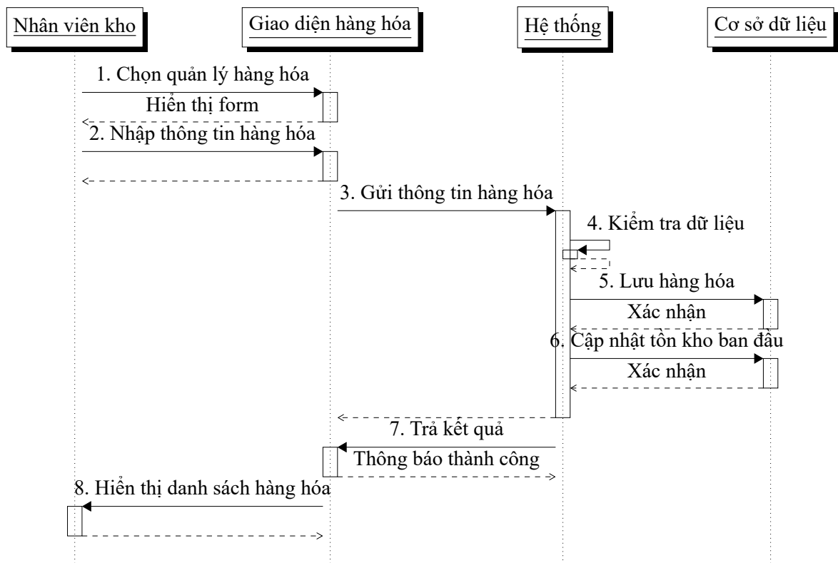
Hình 5.2: Sequence diagram UC13 – Thêm hàng hóa
