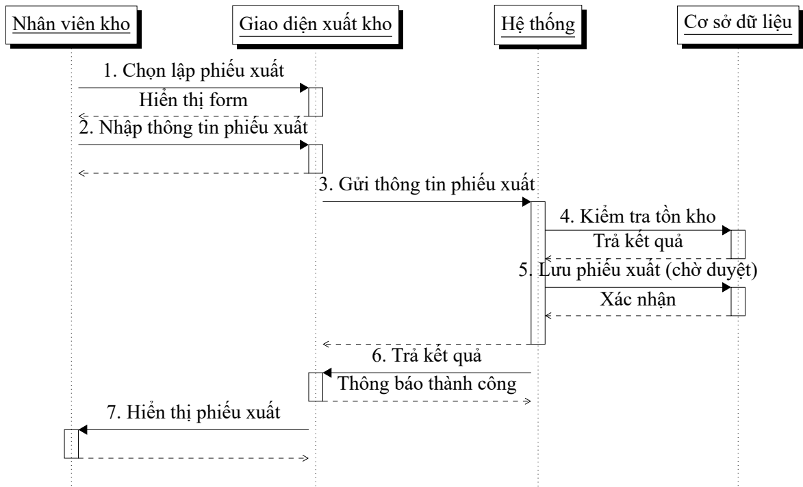
Hình 5.5: Sequence diagram UC28 – Lập phiếu xuất kho
