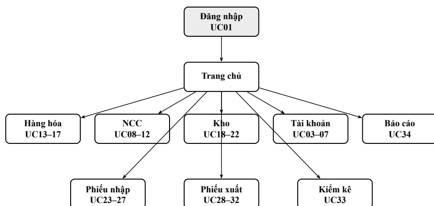
Hình 7.1: Sơ đồ điều hướng màn hình chính (theo use case)
