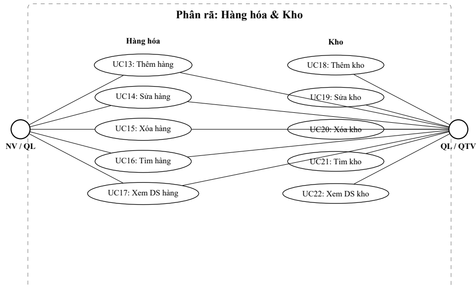
Hình 3.4: Use case phân rã – Hàng hóa (UC13–17) và Kho (UC18–22)
