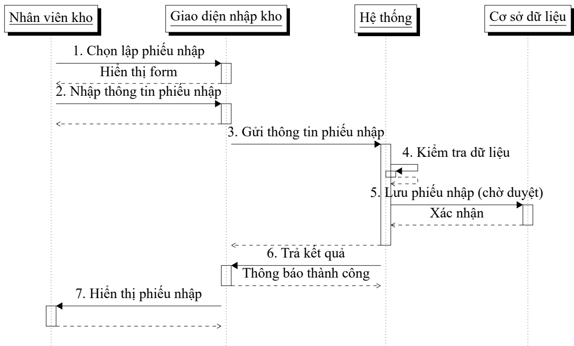
Hình 5.4: Sequence diagram UC23 – Lập phiếu nhập kho
