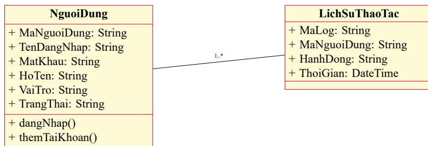
Hình 4.4: Class trong UC03–UC07 – Quản lý tài khoản
