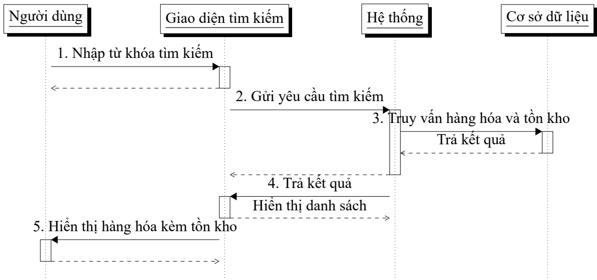
Hình 5.3: Sequence diagram UC16 – Tìm kiếm hàng hóa
