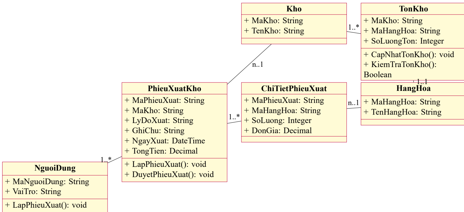
Hình 4.7: Biểu đồ lớp trong ca sử dụng UC28 – Lập phiếu xuất kho
